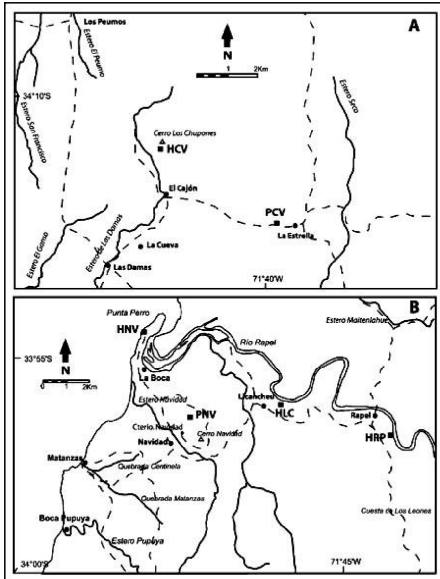
FIG. 3. Mapas con la localización de los estratotipos de las Formaciones Navidad, Licancheu, Rapel y La Cueva. Las líneas punteadas representan las principales carreteras y caminos. A. área de La Estrella. HCV: Holoestratotipo de la Formación La Cueva. PCV: Paraestratotipo de la
