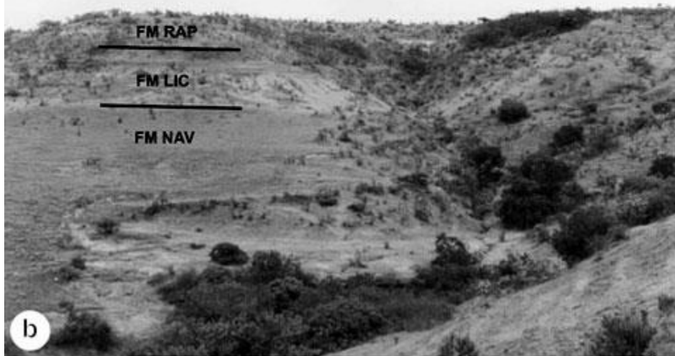
FIG. 5. Fotos de los estratotipos de base y techo de la Formación Navidad. a. Estratotipo de base (Holostratotipo) en Punta Perro mostrando una sucesión de areniscas y limolitas. La foto corresponde aproximadamente a los 30 m basales de la columna (ver figura 3 para su localización y figura 4 para observar la columna). El conglomerado de base no es visible en la foto y se encuentra en la zona de playa, al oeste del acantilado; b. Estratotipo de techo (Paraestratotipo) situado al norte del cerro Navidad (ver figura 3 para su localización). La foto corresponde a la totalidad de la columna (ver figura 4 ). En este sector se pueden observar las formaciones Navidad (Fm Nav), Licancheu (Fm Lic) y Rapel (Fm Rap).
