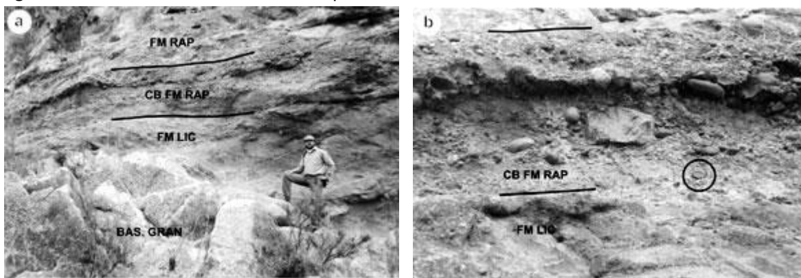
FIG. 6. Foto de la parte basal del estratotipo de la Formación Rapel (Holoestratotipo) situado a unos 500 m de la localidad de Rapel, en la orilla sur del río del mismo nombre (ver figura 3 para su localización y figura 7 para observar la columna). a. De base a techo se pueden observar el basamento granítico (Bas. Gran), la Formación Licancheu (Fm Lic), el conglomerado de base de la Formación Rapel (Cb Fm Rap) y la continuación de la Formación Rapel (Fm Rap). La foto corresponde aproximadamente a los 10 m basales de la columna (ver figura 7); b. Detalle del conglomerado basal de la Formación Rapel. El protector de cámara usado como escala se destaca con un círculo.
