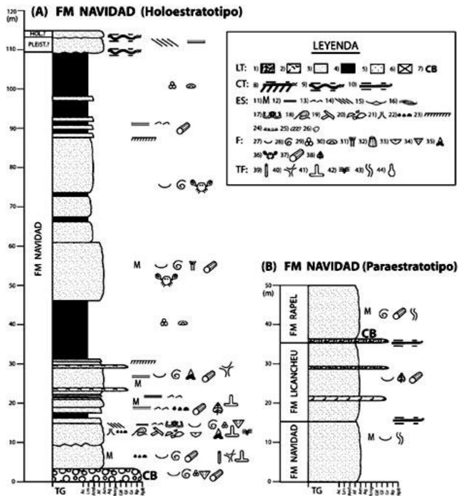
FIG. 4. A. Columna del estratotipo de base (Holostratotipo) de la Formación Navidad; B. Columna del estratotipo de techo (Paraestratotipo) de la Formación Navidad (ver figura 3 para localización de las columnas). TG: Tamaño de grano. Ac: arcilla, Lm: Limo, Amf: arena muy fina, Af: arena fina, Am: arena media, Ag: arena gruesa, Amg: arena muy gruesa, Glf: gravilla fina, Gf: gravilla, Gr: grava, Rp: ripio, Rpb: Ripio de bolones, LT: Litología. 1. conglomerado, 2. coquina, 3. arenisca, 4. lutita y limolita, 5. granito, 6. tramo cubierto, 7. conglomerado basal de la unidad. CT: Tipo de contacto entre unidades. 8. discordancia, 9. disconformidad, 10. paraconformidad. ES: Estructuras sedimentarias. 11. estructura maciza, 12. laminación paralela, 13. ondulitas asimétricas, 14.
