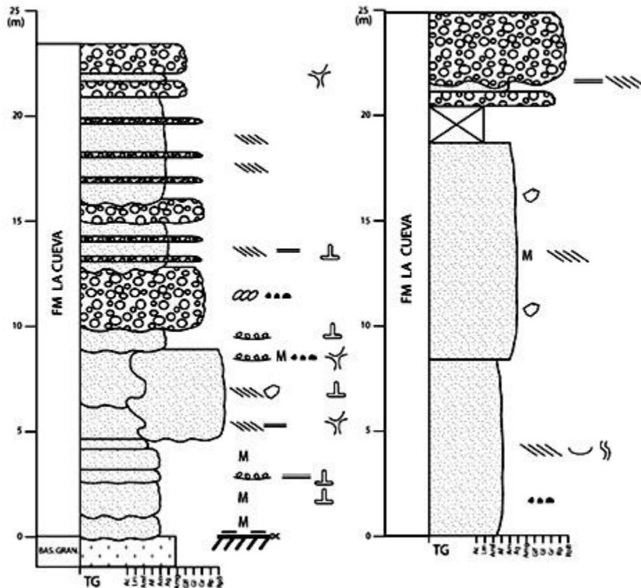
(A) FM LA CUEVA (Paraestratotipo) (B) FM LA CUEVA (Holoestratotipo)
